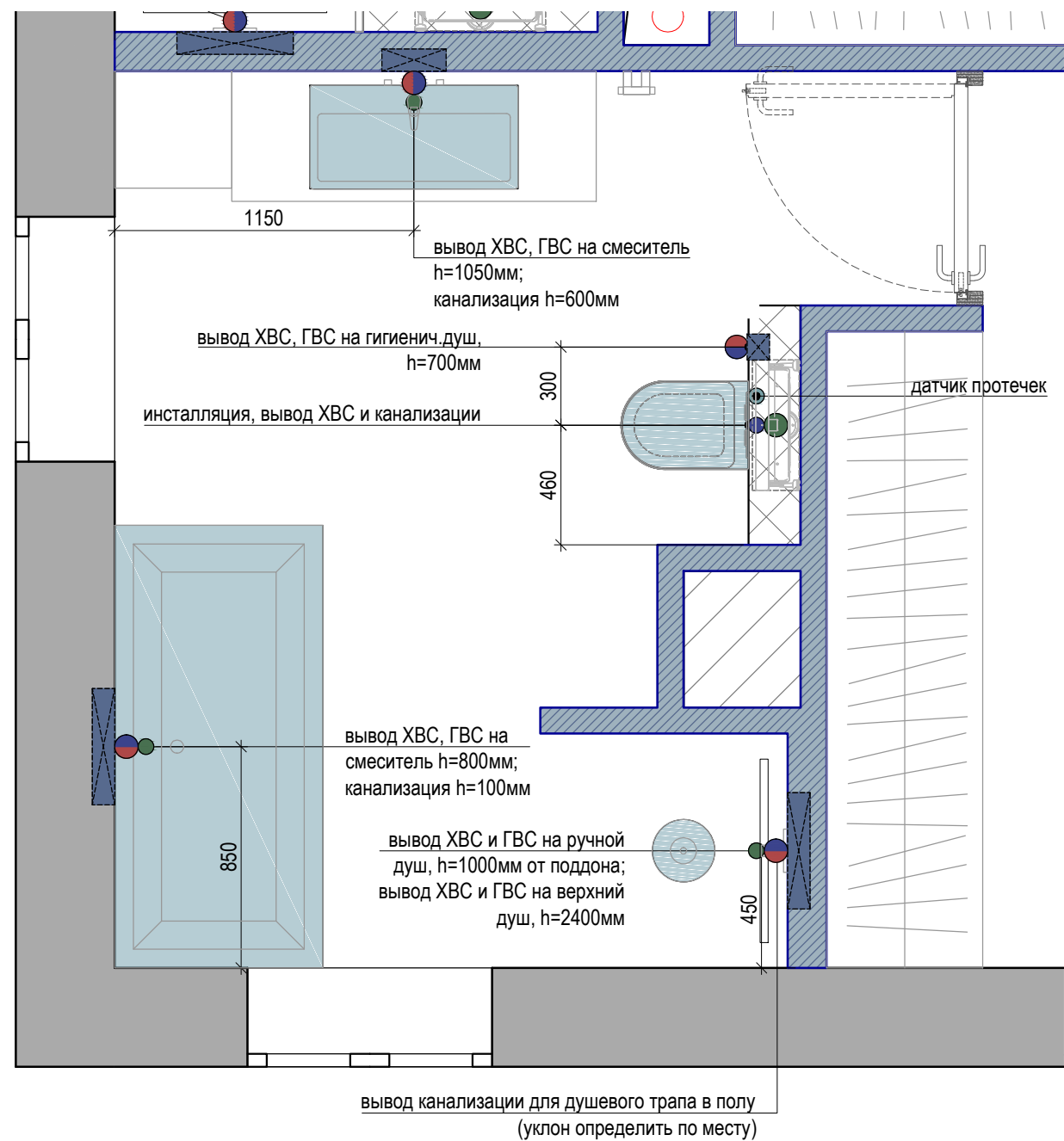
План привязки сантехнического оборудования. Сан. узел, 2 этаж
