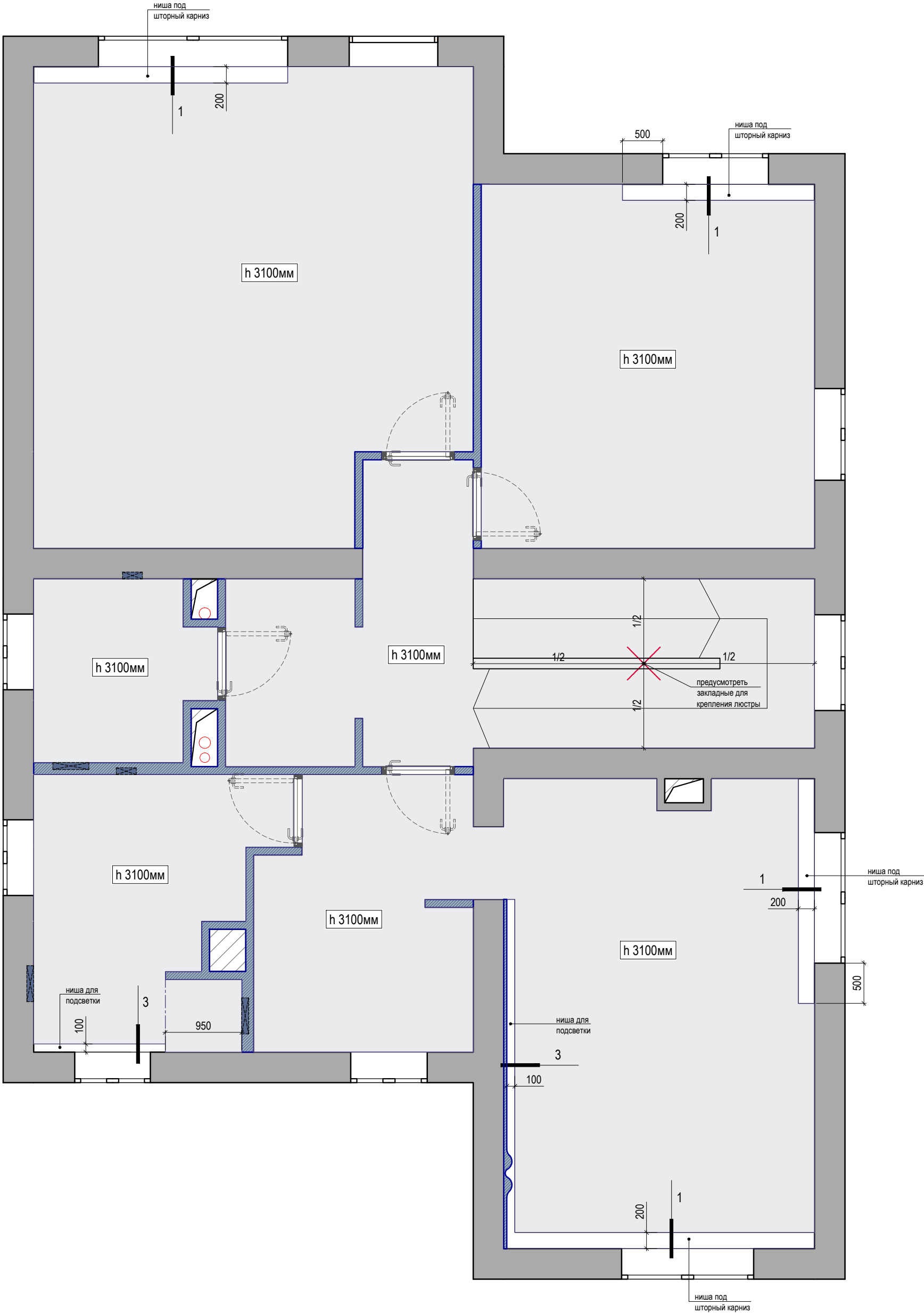
План потолков с указанием высотных отметок. 2 этаж
