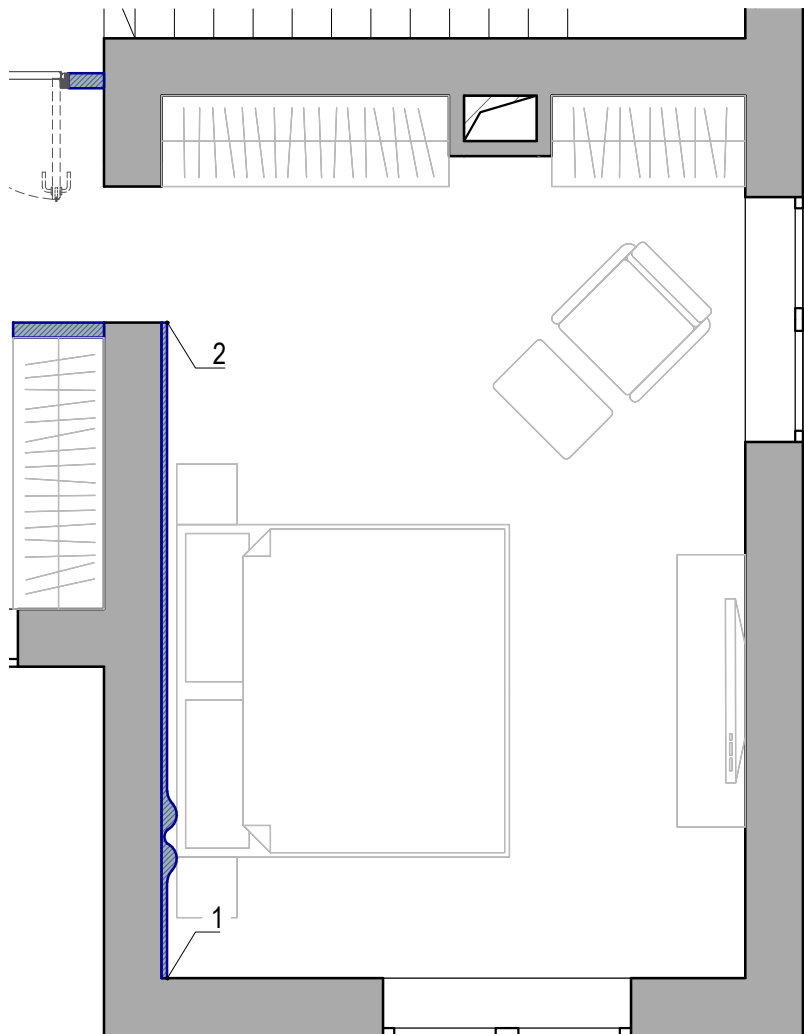
План маяков для разверток стен
