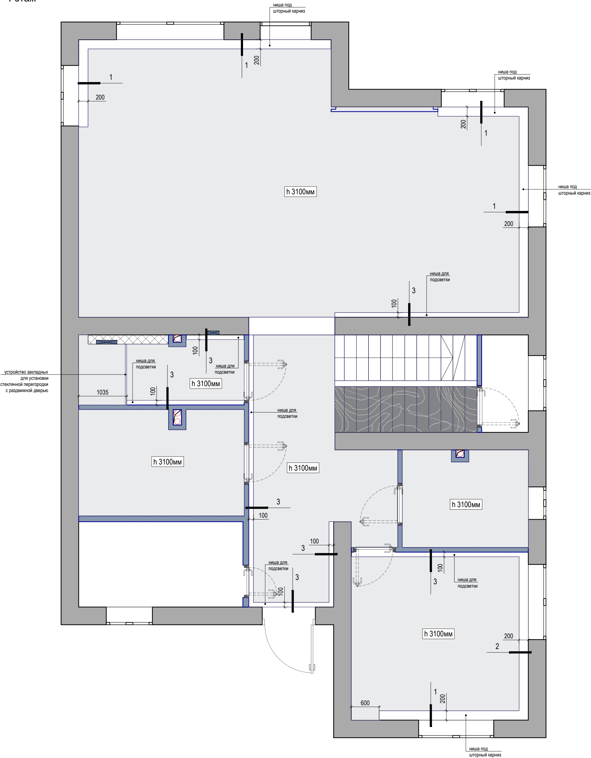
План потолков с указанием высотных отметок. 1 этаж
