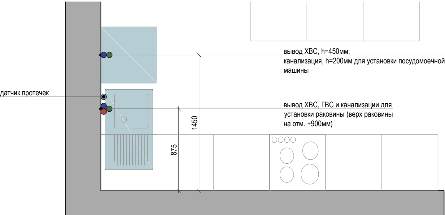
План привязки сантехнического оборудования. Кухня, 1 этаж
