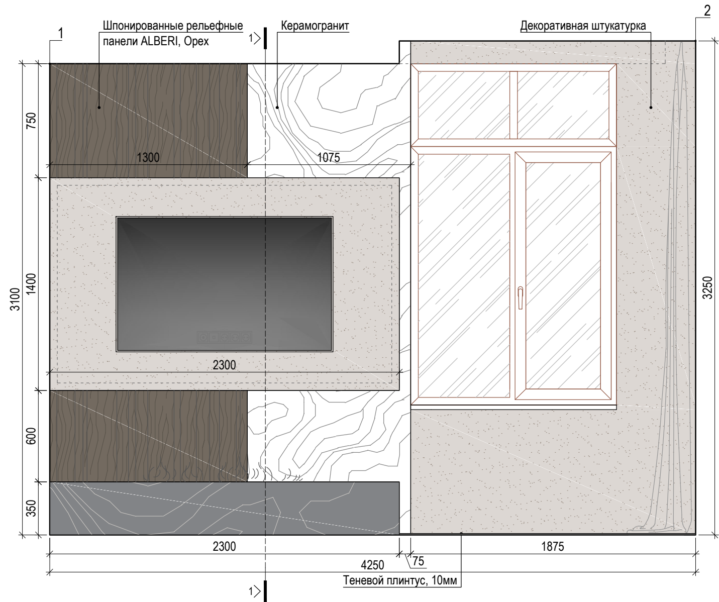
Развертка стены гостиной
