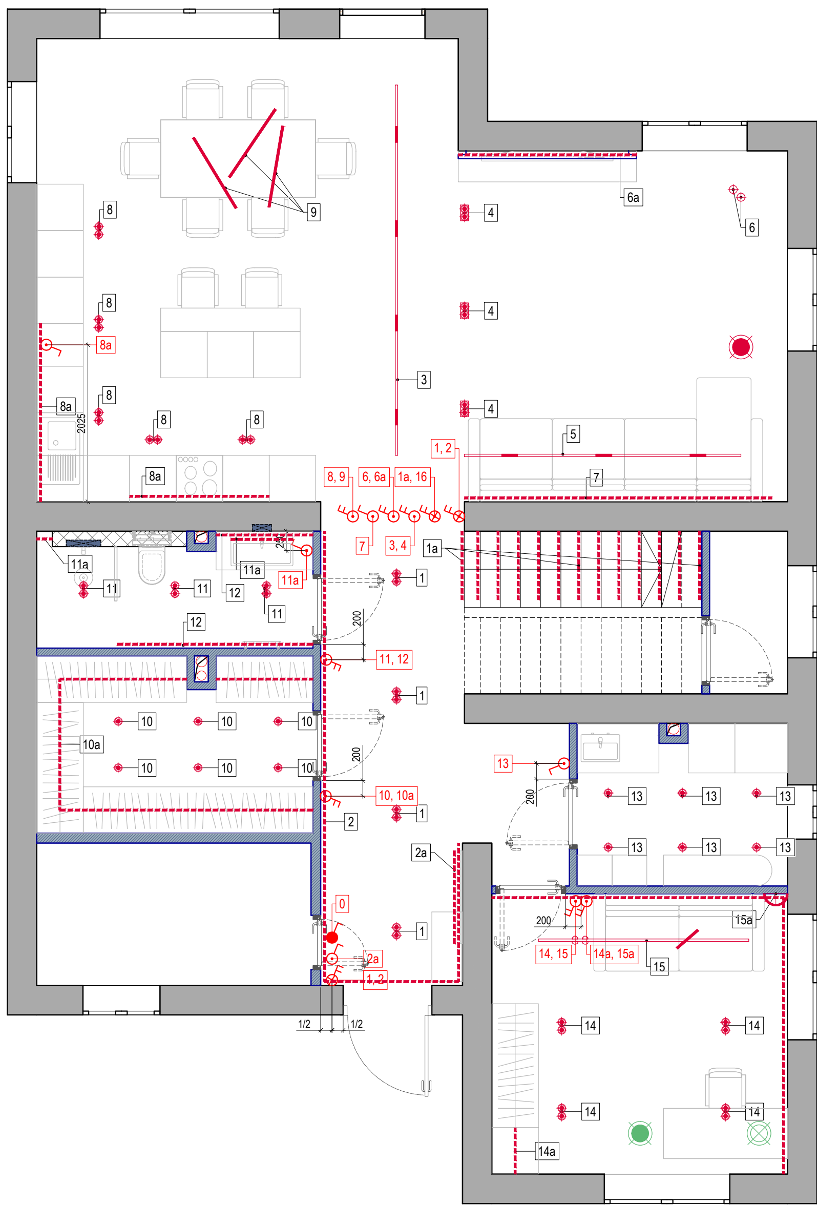
План привязки выключателей с указанием групп включения светильников. 1 этаж
