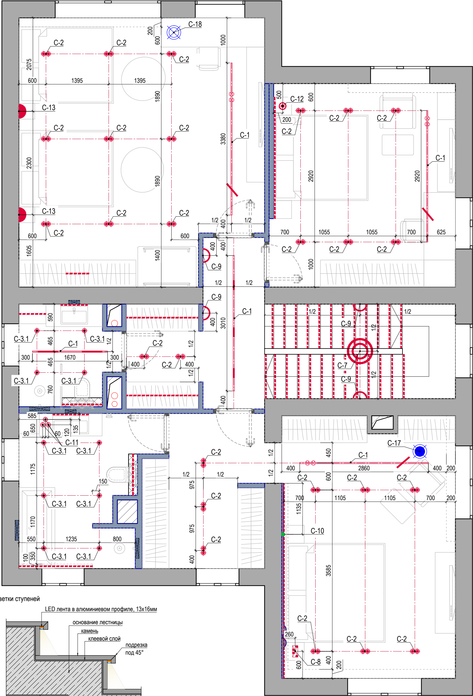
План привязки осветительного оборудования. 2 этаж
