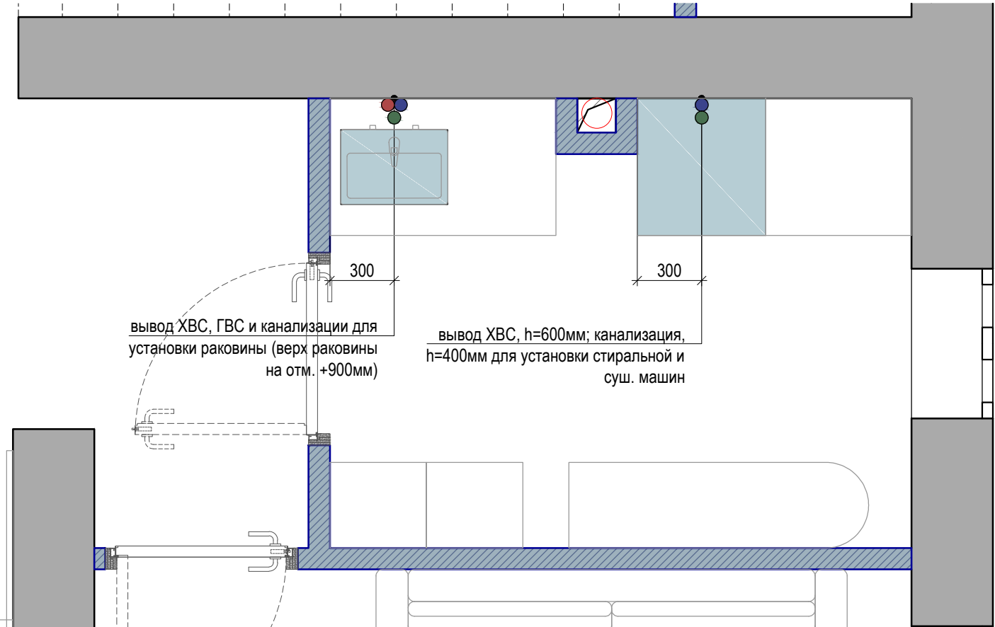
План привязки сантехнического оборудования. Постирочная, 1 этаж
