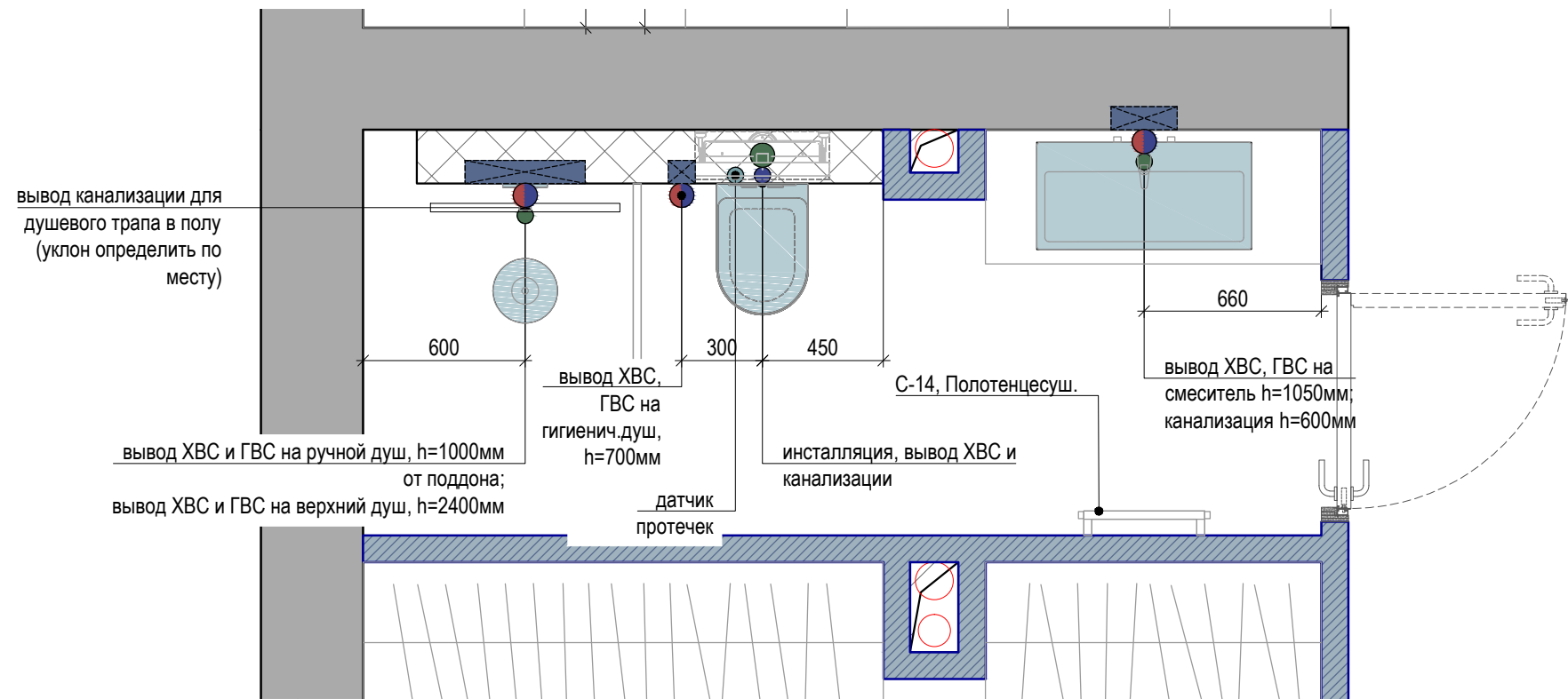
План привязки сантехнического оборудования. Сан. узел, 1 этаж
