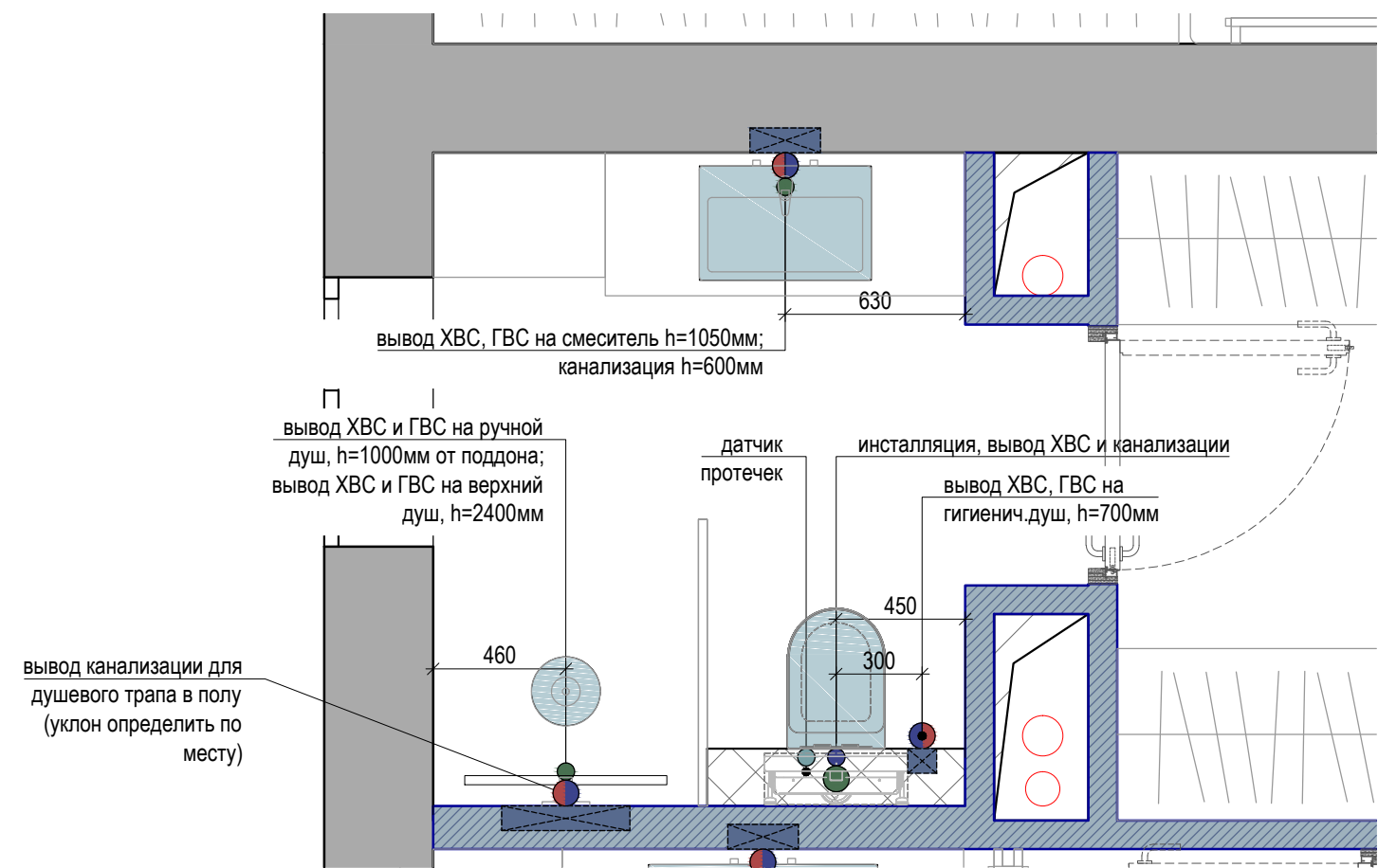
План привязки сантехнического оборудования. Сан. узел, 2 этаж
