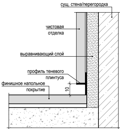
Узел устройства тенового плинтуса
