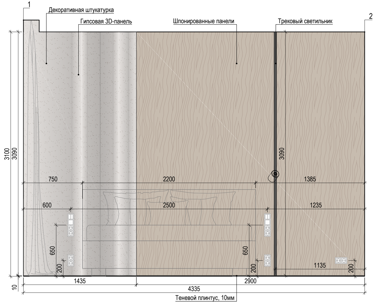
Развертка стены спальни
