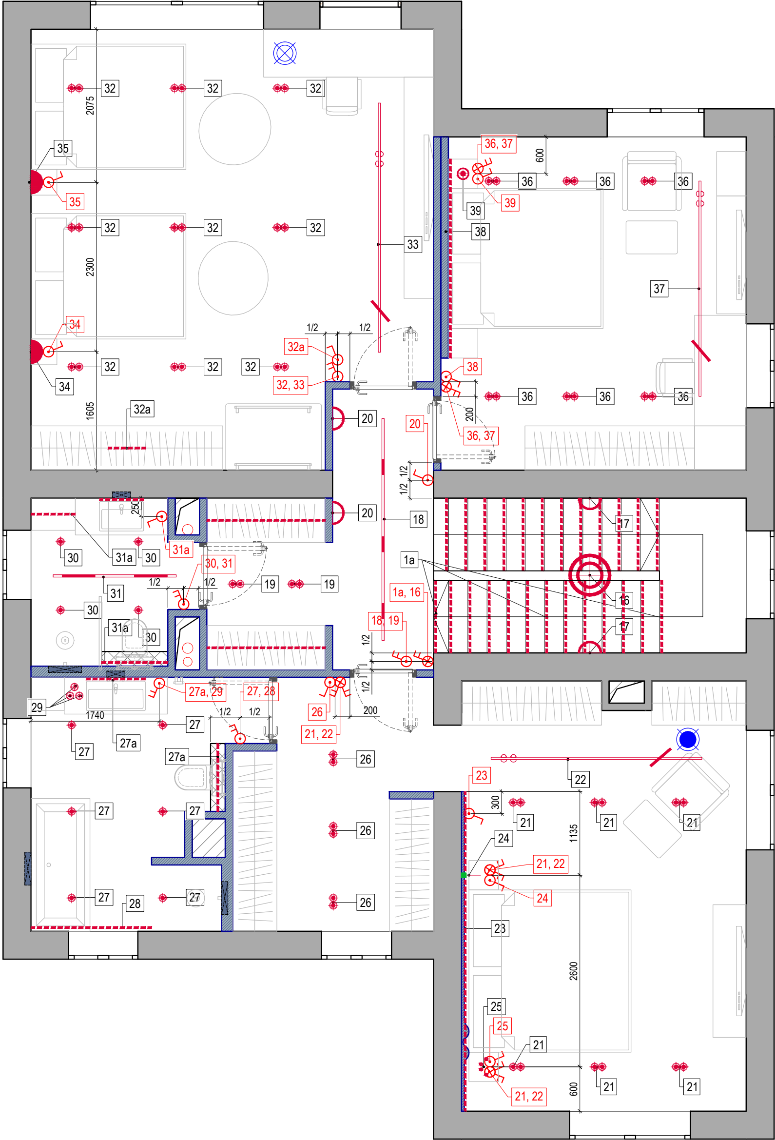
План привязки выключателей с указанием групп включения светильников. 2 этаж
