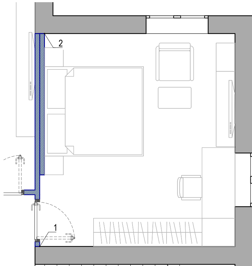
План маяков для разверток стен
